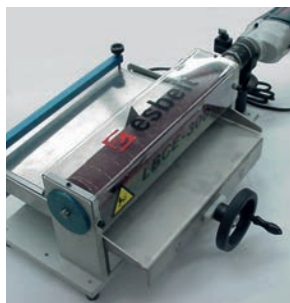
Detalle de la biseladora con el taladro colocado
